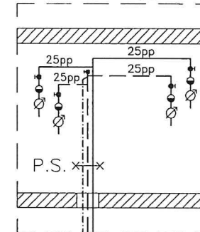
Schemat Pionopiętra
